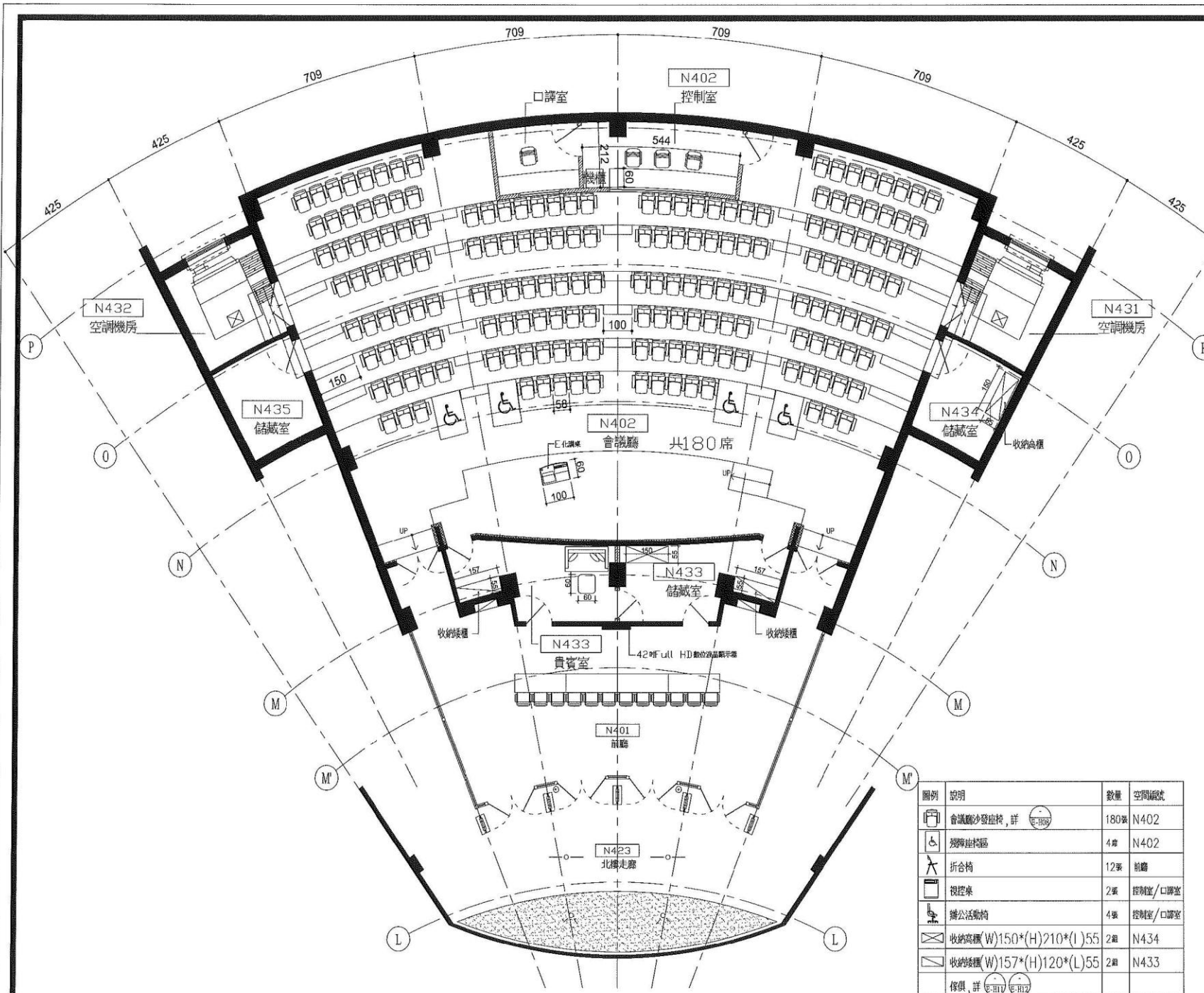
1 國際會議廳座椅及傢俱平面配置圖 S:1/120
